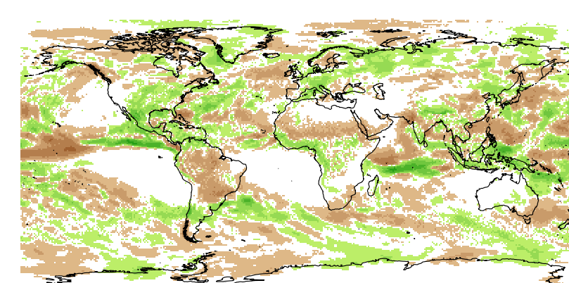
Sep totprec
