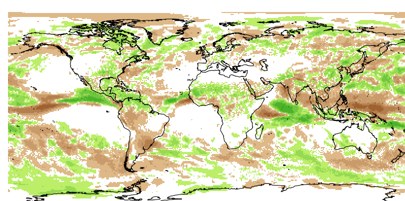
Aug totprec
