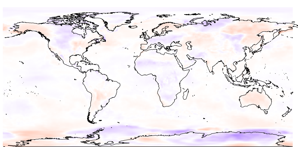
May totprec
