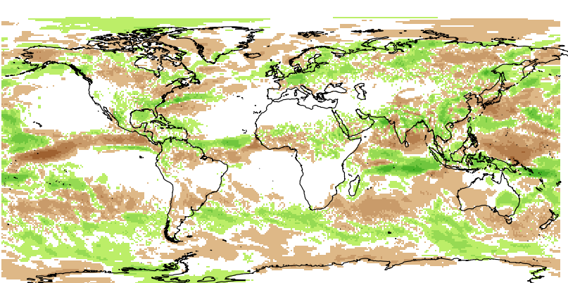
Jul totprec
