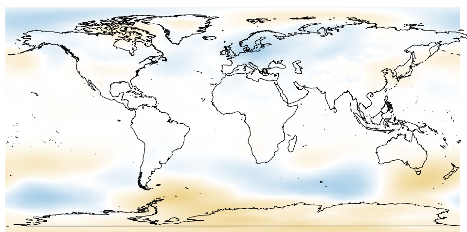
Jul slp
