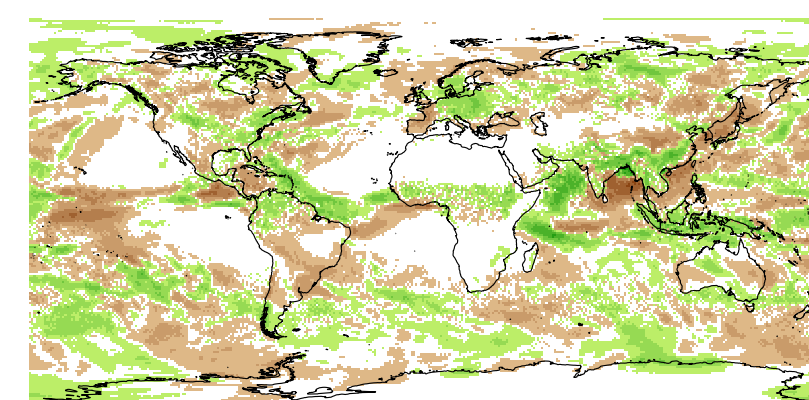
Jun totprec
