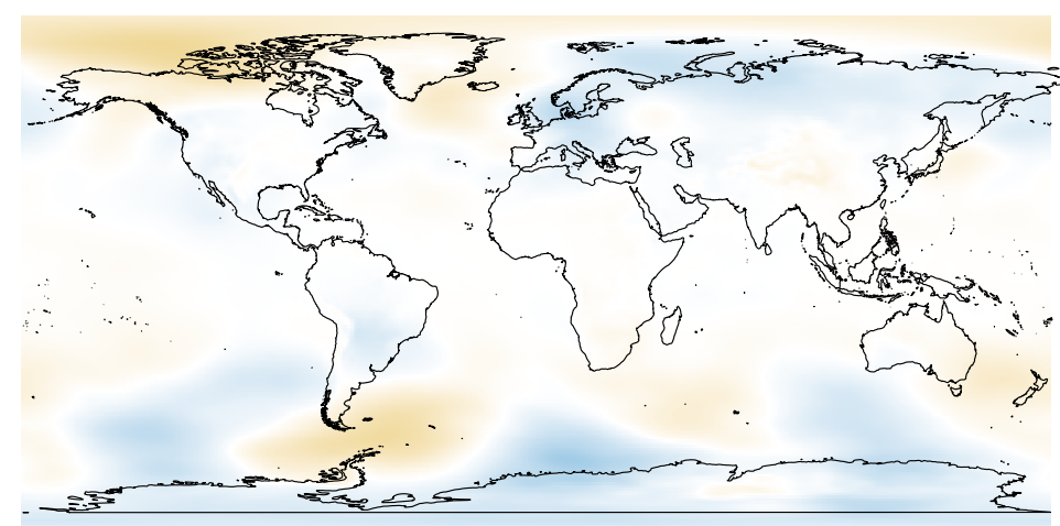
Sep slp
