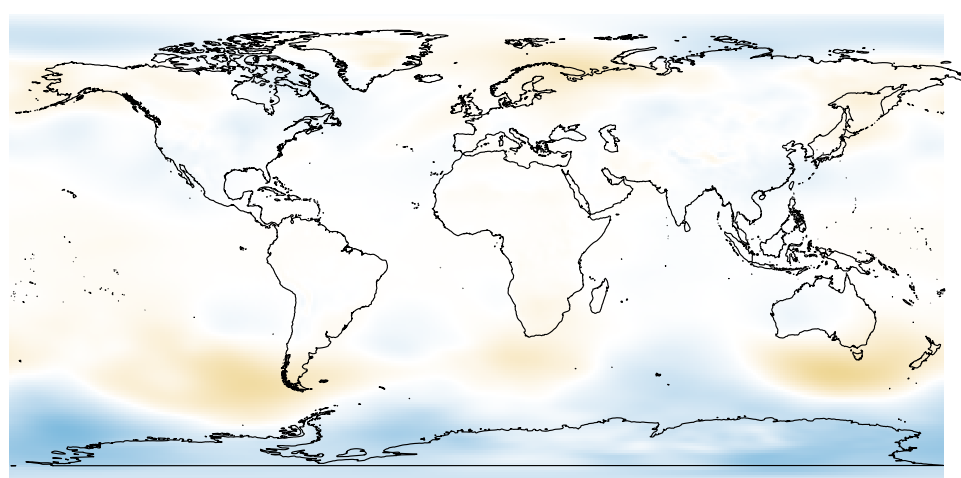
Aug slp
