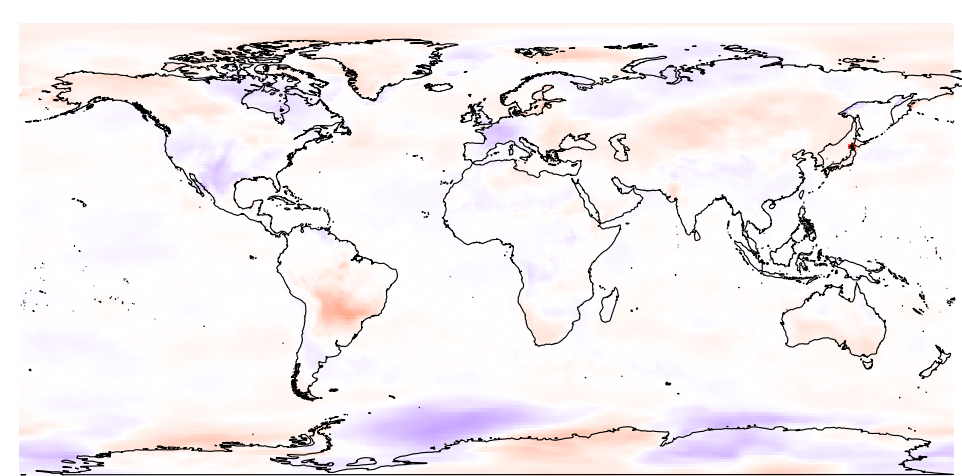
Jun totprec
