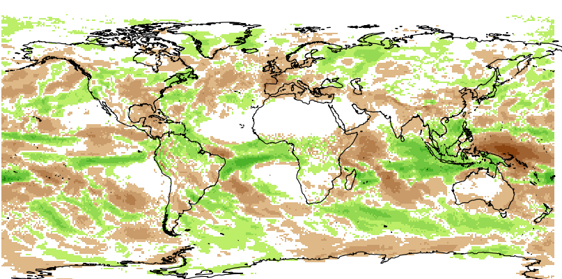
Apr totprec
