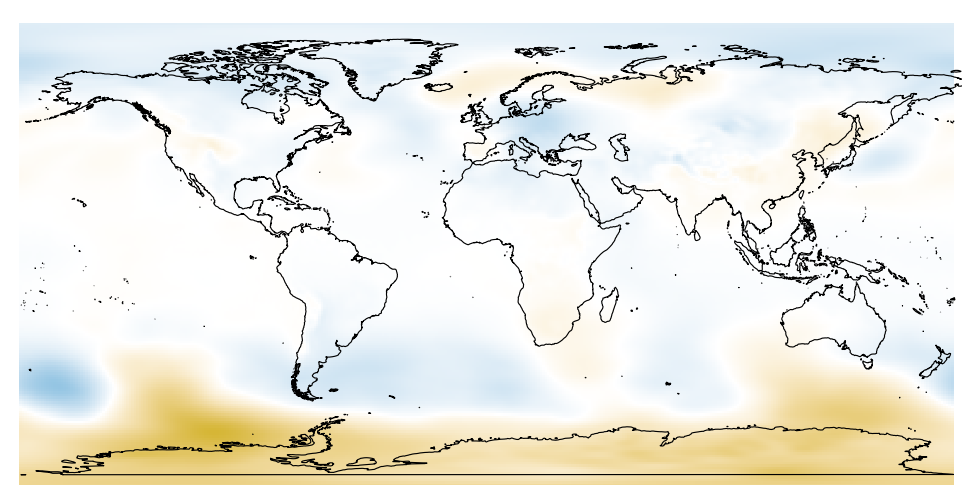
Jun slp
