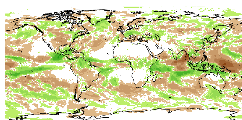
May totprec
