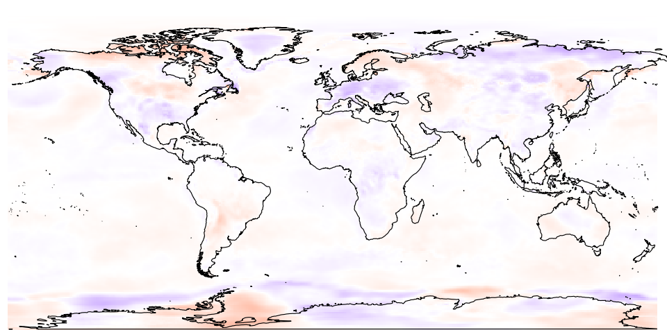
Apr totprec
