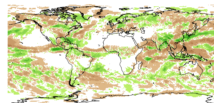
Jun totprec
