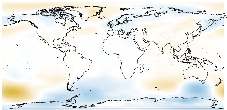
Jul slp
