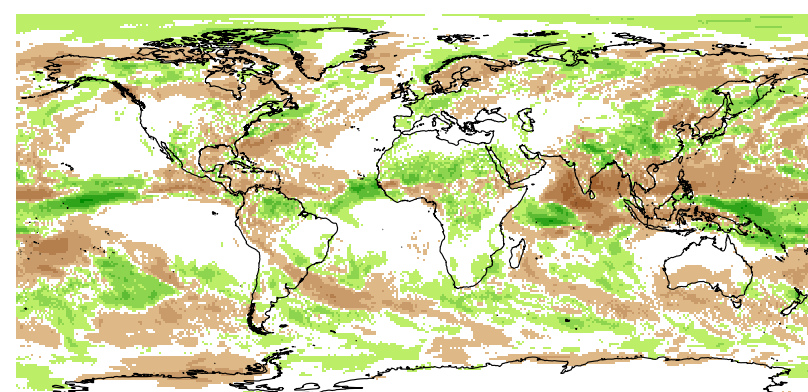
Aug totprec
