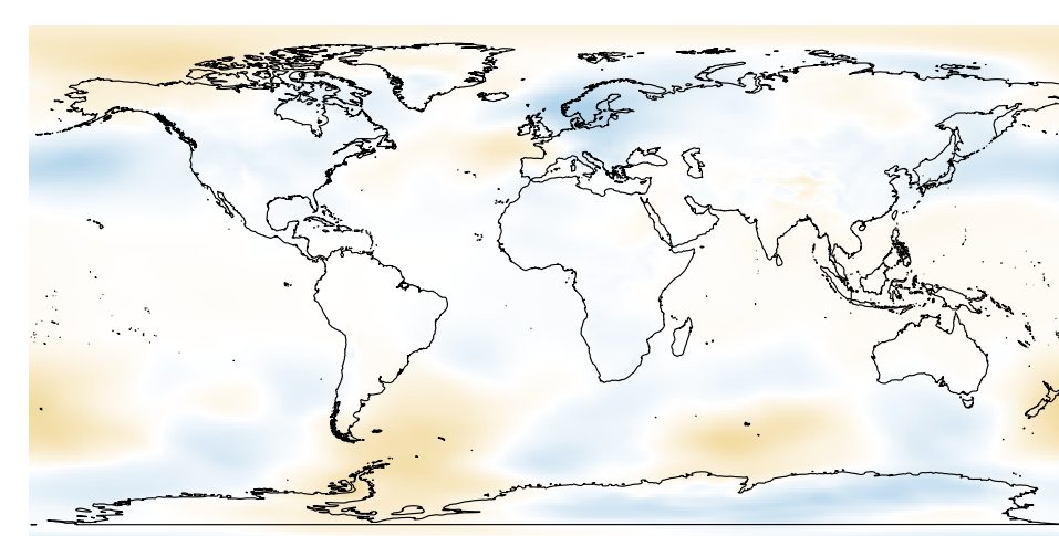
Jun slp
