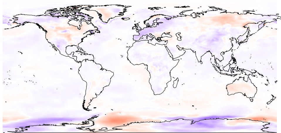
Apr totprec
