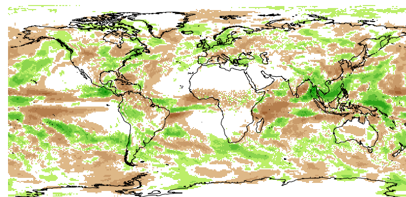
May totprec
