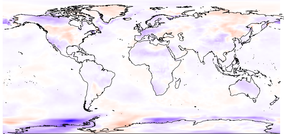
May totprec
