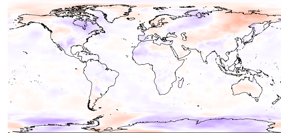
Jun totprec
