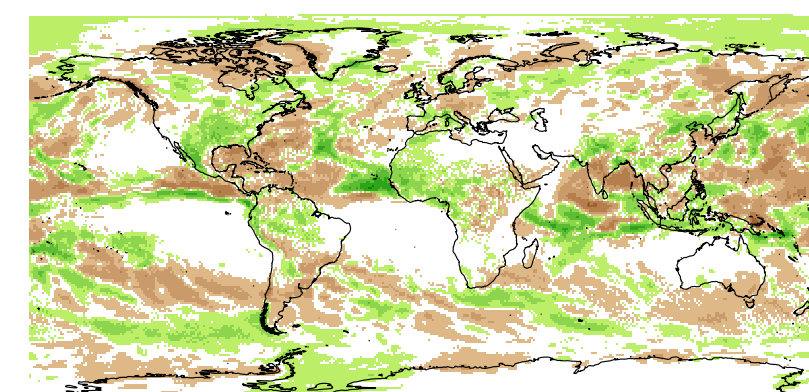
Sep totprec
