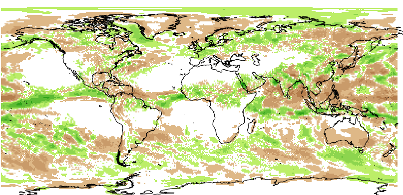
Jul totprec
