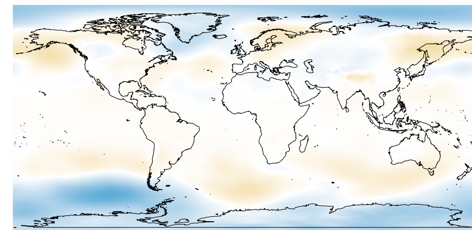
Sep slp
