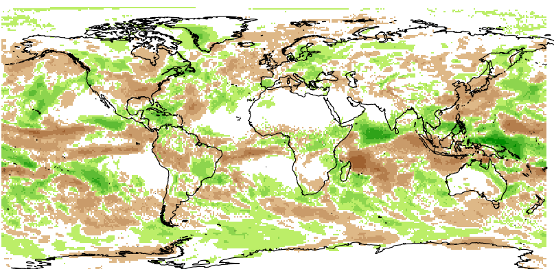
Apr totprec
