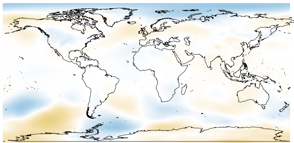
Aug slp
